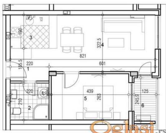
основа I спрата
